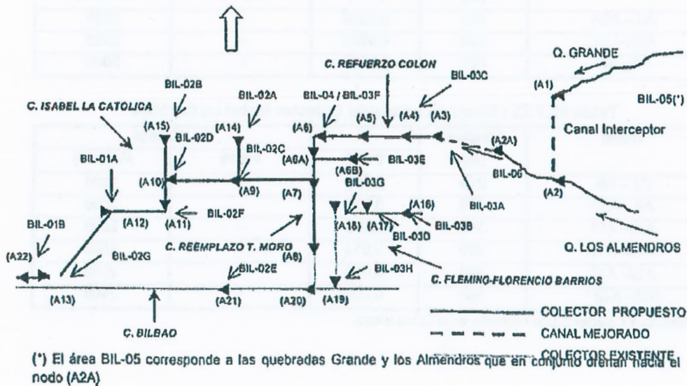
Figura VII.7.7 : Esquema Solución Quebrada de Apoquindo
